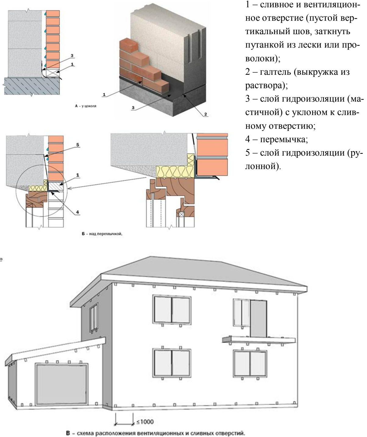
Рис. 14. Меры по отводу конденсата из зоны потенциального увлажнения
