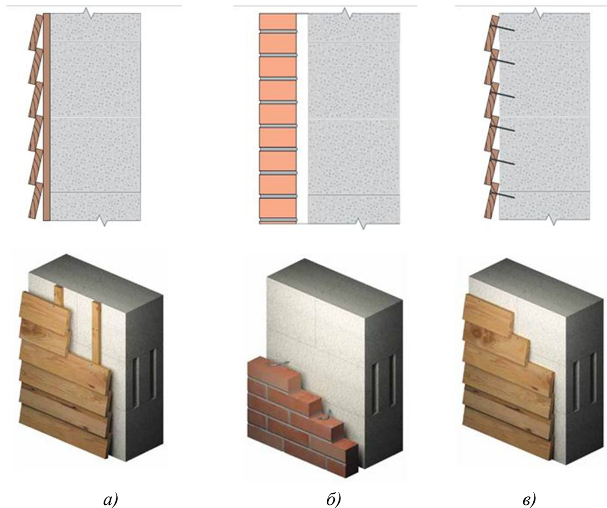
Рис. 9. Облицовка на отnose: а — крепление облицовочных изделий к направляющим; б — облицовка кладкой из штучных материалов; в — механическое крепление штучных материалов к кладке
