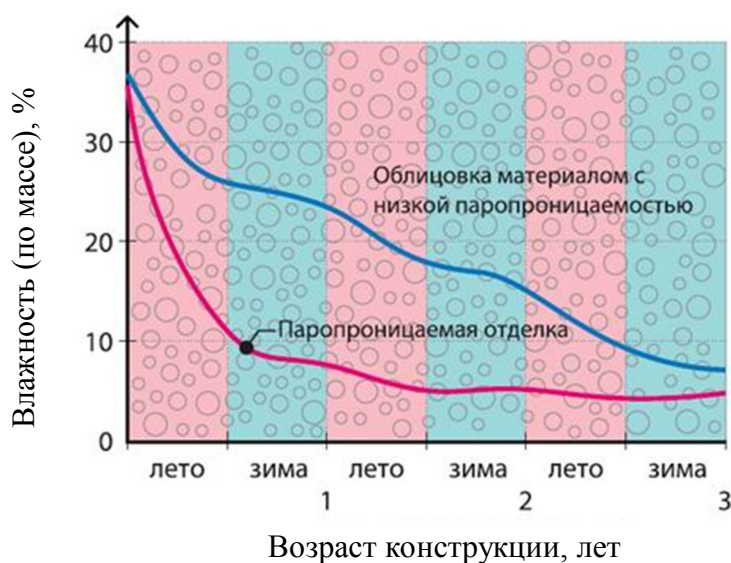
Рис. 8. Высыхание газобетона в однослойных конструкциях
