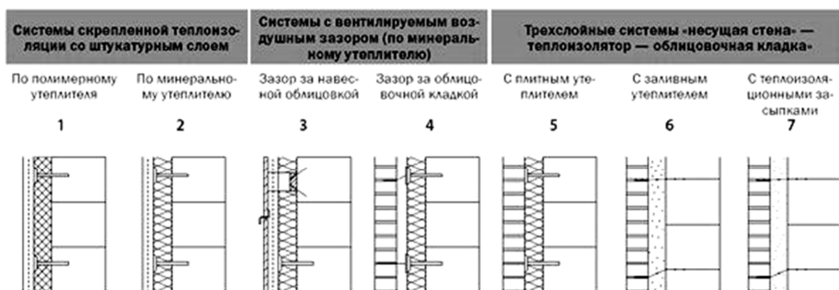
Рис. 20. Системы теплоизоляции
