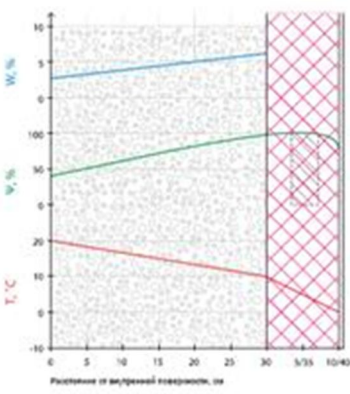
B1 – мокрое утепление по ППС 50/100 мм
