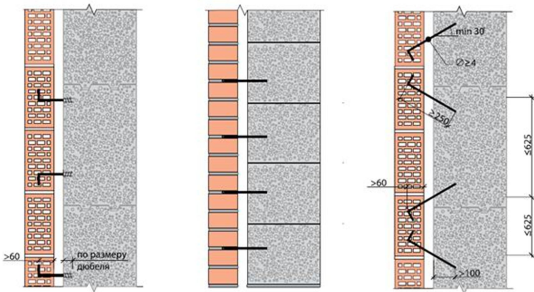
Рис. 16. Связь облицовочного и основного слоев кладки:
