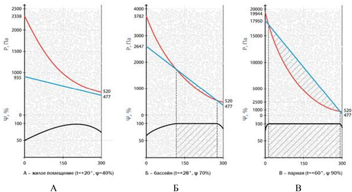
Рис. 26. Влияние микроклимата на распределение влажности воздуха в порах по толщине стены: А – жилое помещение ( t = 20^\circ , \psi = 40\% ); Б – бассейн ( t = 28^\circ , \psi = 70\% ); В – баня ( t = 60^\circ , \psi = 90\% ).
